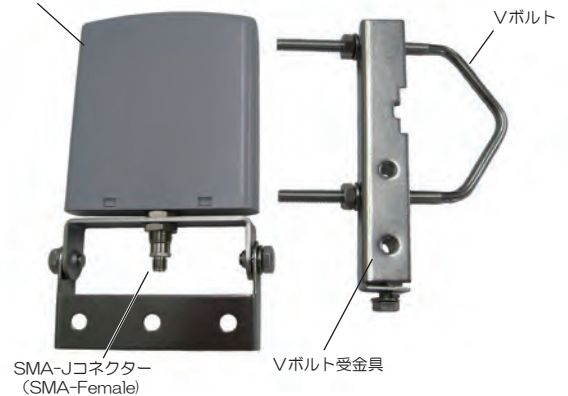
アンテナ (PA0509SU)
