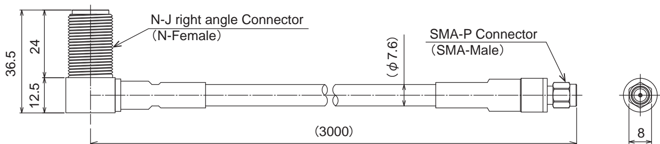
■ 外観図
