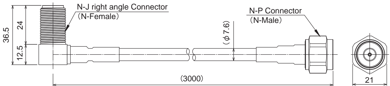
■ 外観図
